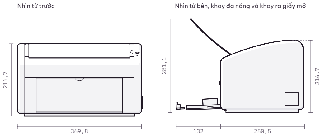
Hình 8-1 · Kích thước tính bằng mm: rộng 369,8 · sâu 250,5 (thêm 132 khi mở khay đa năng) · cao 216,7 (281,1 khi mở khay ra giấy)
